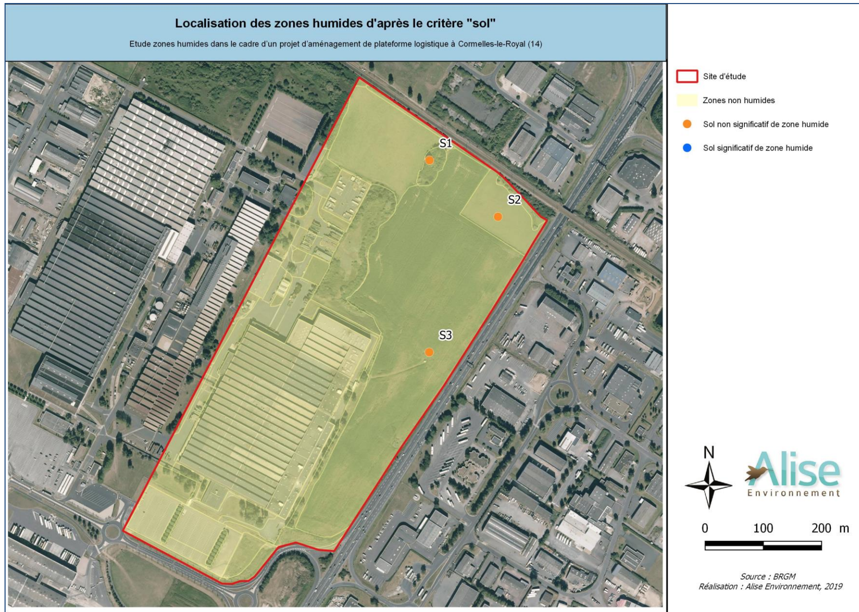
Figure 8 : Zones humides définies par le critère « sol »
