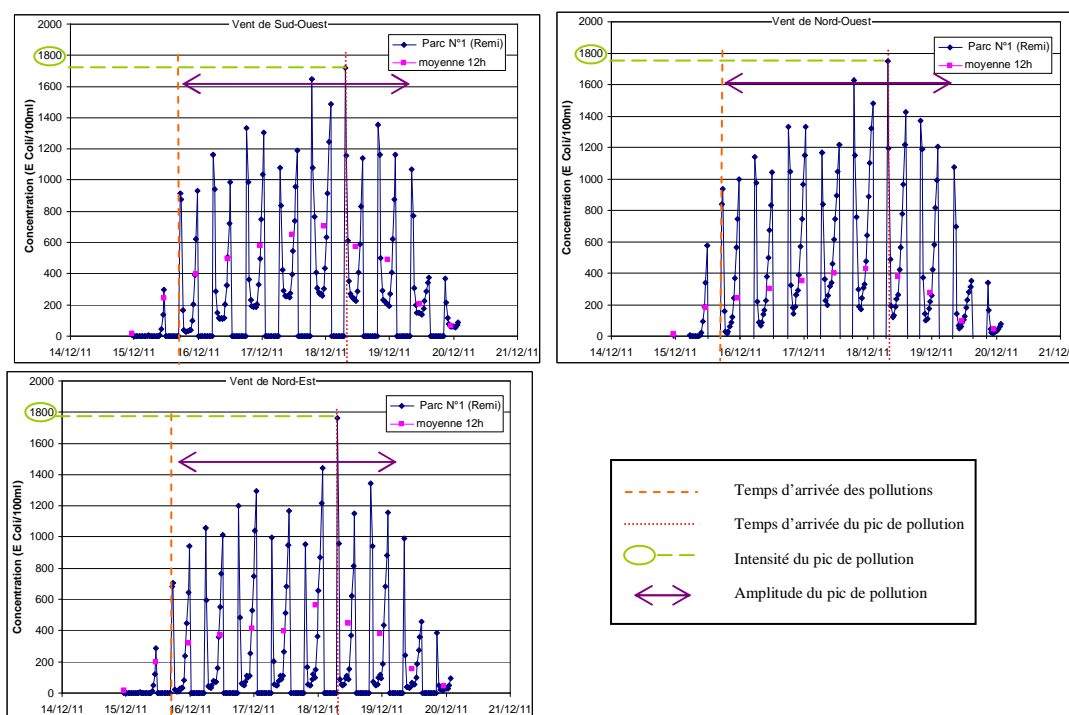
Figure 3-12 : Chroniques temporelles des concentrations dans l'eau de la zone classée 14-170 pour différentes conditions de vent et en temps de pluie semestrielle hivernal
